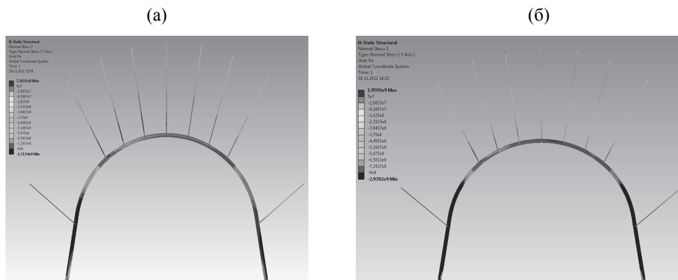
Рис. 2. Эпюры вертикальных напряжений бурманной и анкерной крепи: при расстоянии 14 м от груди очистного забоя до выработки (а); грудь очистного забоя сравнялась с вертикальной осью симметрии выработки (б)
