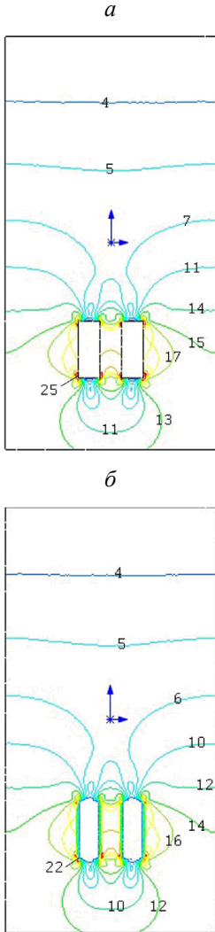
Рис. 1. Ізолінії напружень: а – порожні камери, б – камери із закладкою; 4, 5, 6 – 25 – максимальні стискні напруження, МПа
