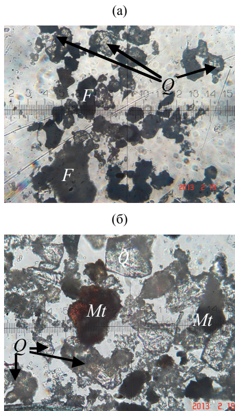
Рис. 1. Микрофотография продуктов разрушения гранитов (а) и железистых кварцитов (б); увеличение 300×: Q – кварц, F – полево шпат, Mt – магнетит
