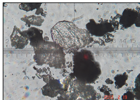
Рис. 2. Микрофотография продуктов железистого кварцита обработанного насыщенным раствором Na_2CO_3 увеличение 300×: светлые зерна – кварц, темные – магнетит
